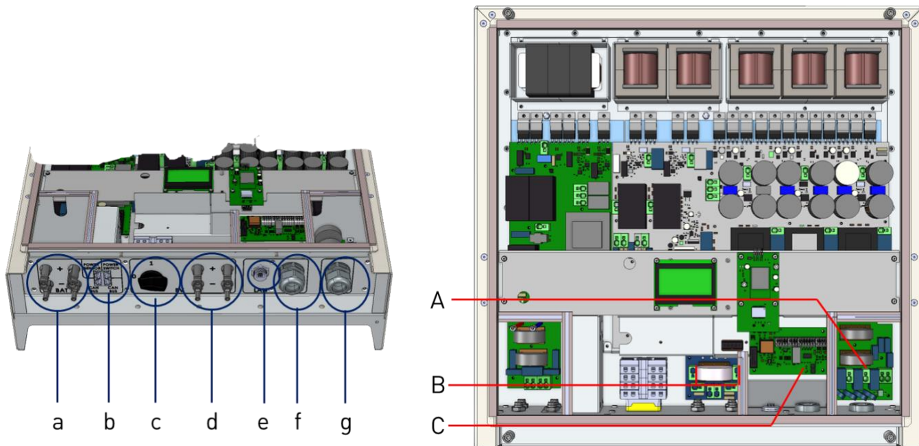
Obr. 5-1 Přehled konektorového oddílu a vnitřních propojovacích prvků
