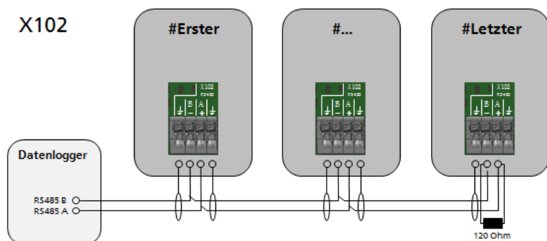
Obr. 6-3 Připojení datového záznamníku
