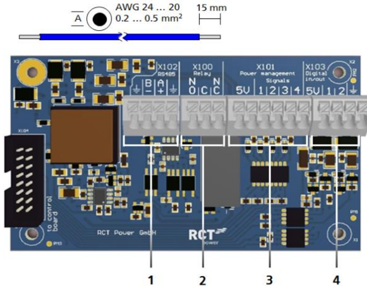
Obr. 6-1 Deska vstupů/výstupů
