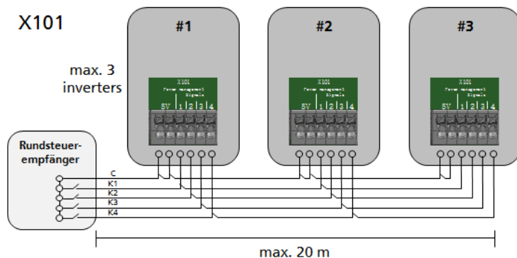
Obr. 6-5 Připojení přijímače HDO
