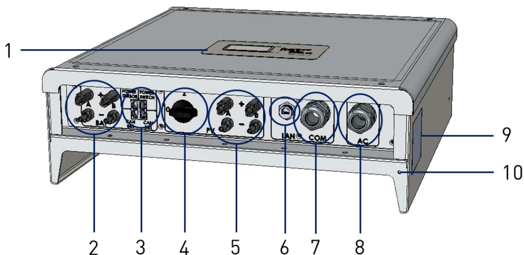
Obr. 3-3 Popis produktu
