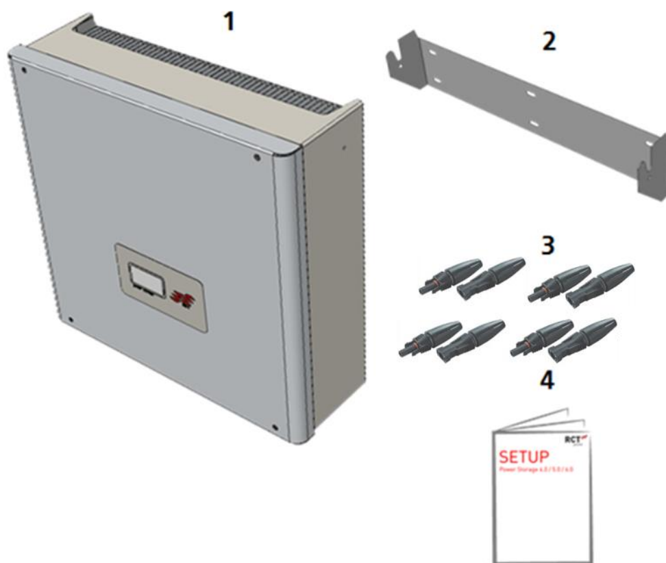
Obr. 3-2 Rozsah dodávky
