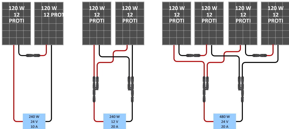
Příklady z série, paralelní a série/paralelní sluneční pole.
