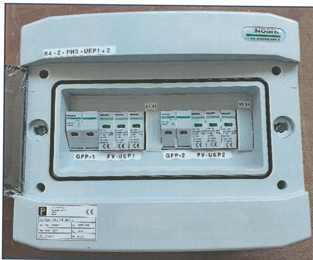
Obr. 3 - Rozváděč R4-2-PHS-UEP1+2 (otevřený)
