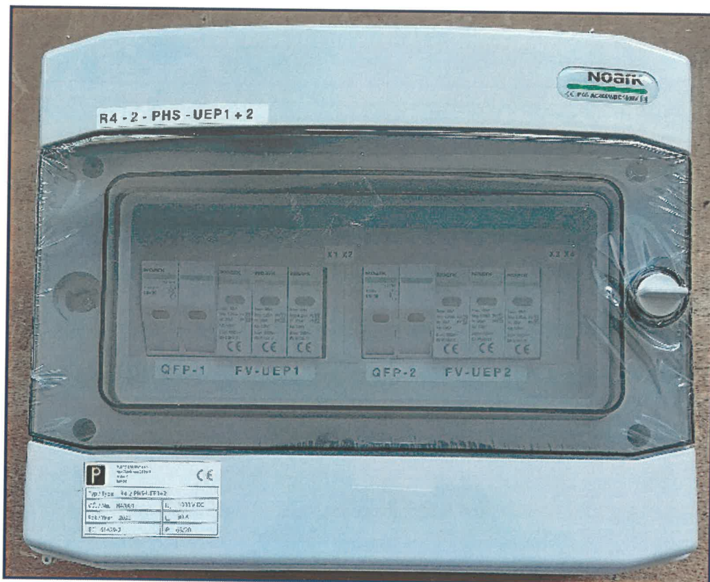
Obr. 2 - Rozváděč R4-2-PHS-UEP1+2
