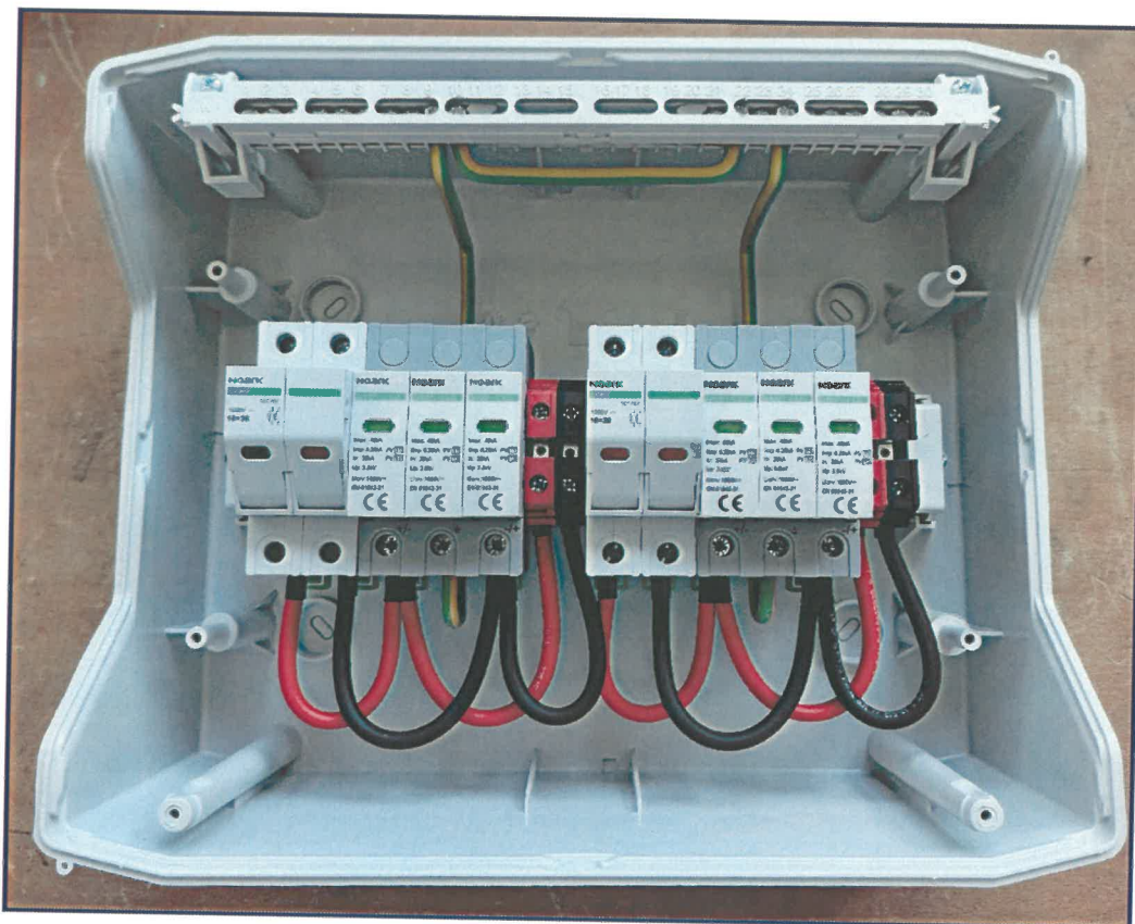
Obr. 4 - Vybavení rozváděče R4-2-PHS-UEP1+2
