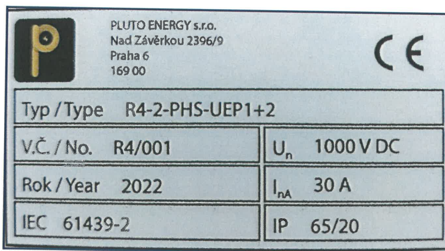
Obr. 1 - Výrobní štítek
