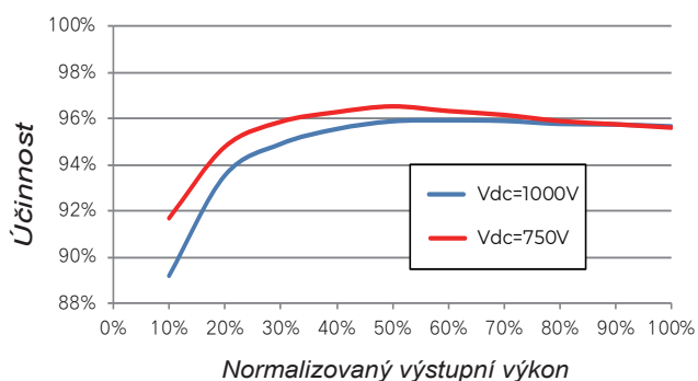
Křivka účinnosti
