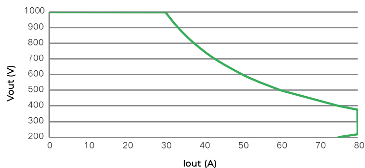
Křivka výstupního napětí a výstupního proudu
